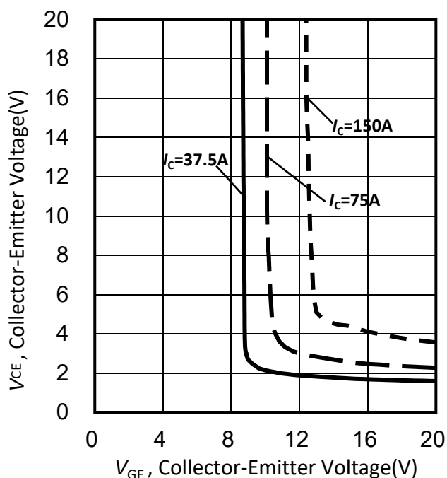
Figure 12. 典型 V_{CE(sat)}-V_{GE(th)} 特性曲线/Typical V_{CE(sat)}-V_{GE(th)} characteristic( T_{vj}=175^{\circ}\text{C} )
