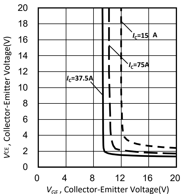
Figure 9. 典型 V_{CE(sat)}-V_{GE(th)} 特性曲线/Typical V_{CE(sat)}-V_{GE(th)} characteristic( T_{vj}=25^{\circ}\text{C} )
