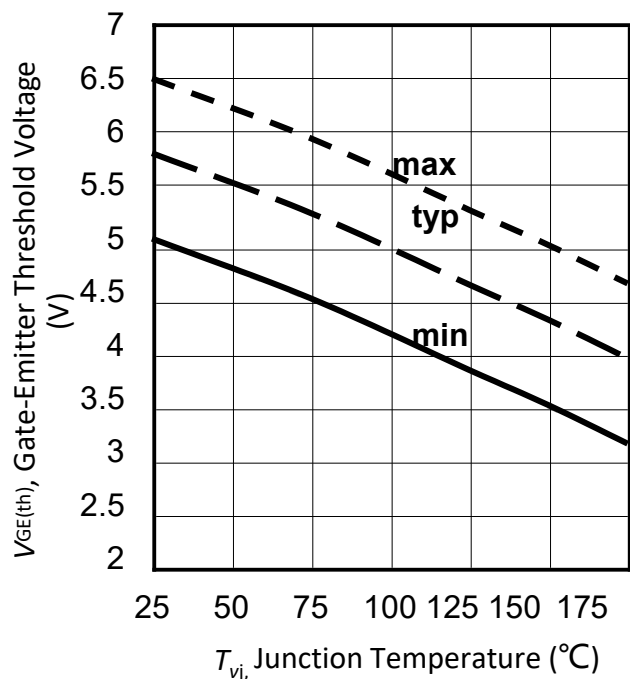
Figure 7. 典型 V_{GE(th)} - T_j 特性曲线/Typical V_{GE(th)} - T_j characteristic ( I_c=2.4mA )
