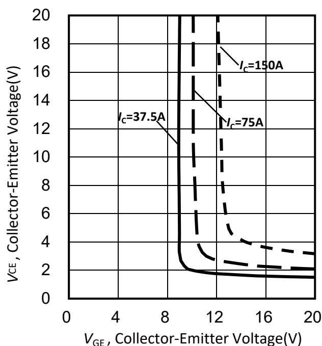
Figure 10. 典型 V_{CE(sat)}-V_{GE(th)} 特性曲线/ Typical V_{CE(sat)}-V_{GE(th)} characteristic( T_{vj}=125^{\circ}\text{C} )
