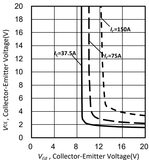
Figure 11. 典型 V_{CE(sat)}-V_{GE(th)} 特性曲线/Typical V_{CE(sat)}-V_{GE(th)} characteristic( T_{vj}=150^{\circ}\text{C} )
