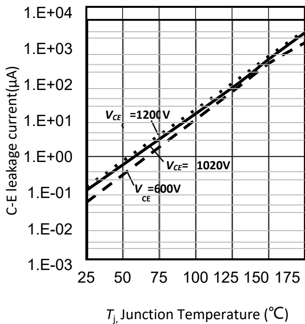
Figure 8. 典型 V_{GE(th)} - T_j 特性曲线/Typical I_{CES} - T_j characteristic ( V_{GE}=0V )
